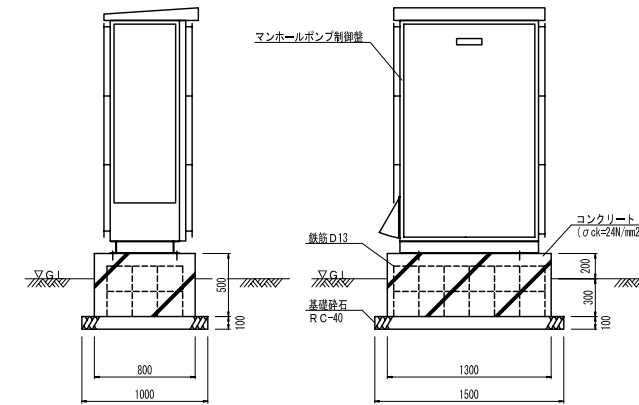
制御盤基礎詳細図
