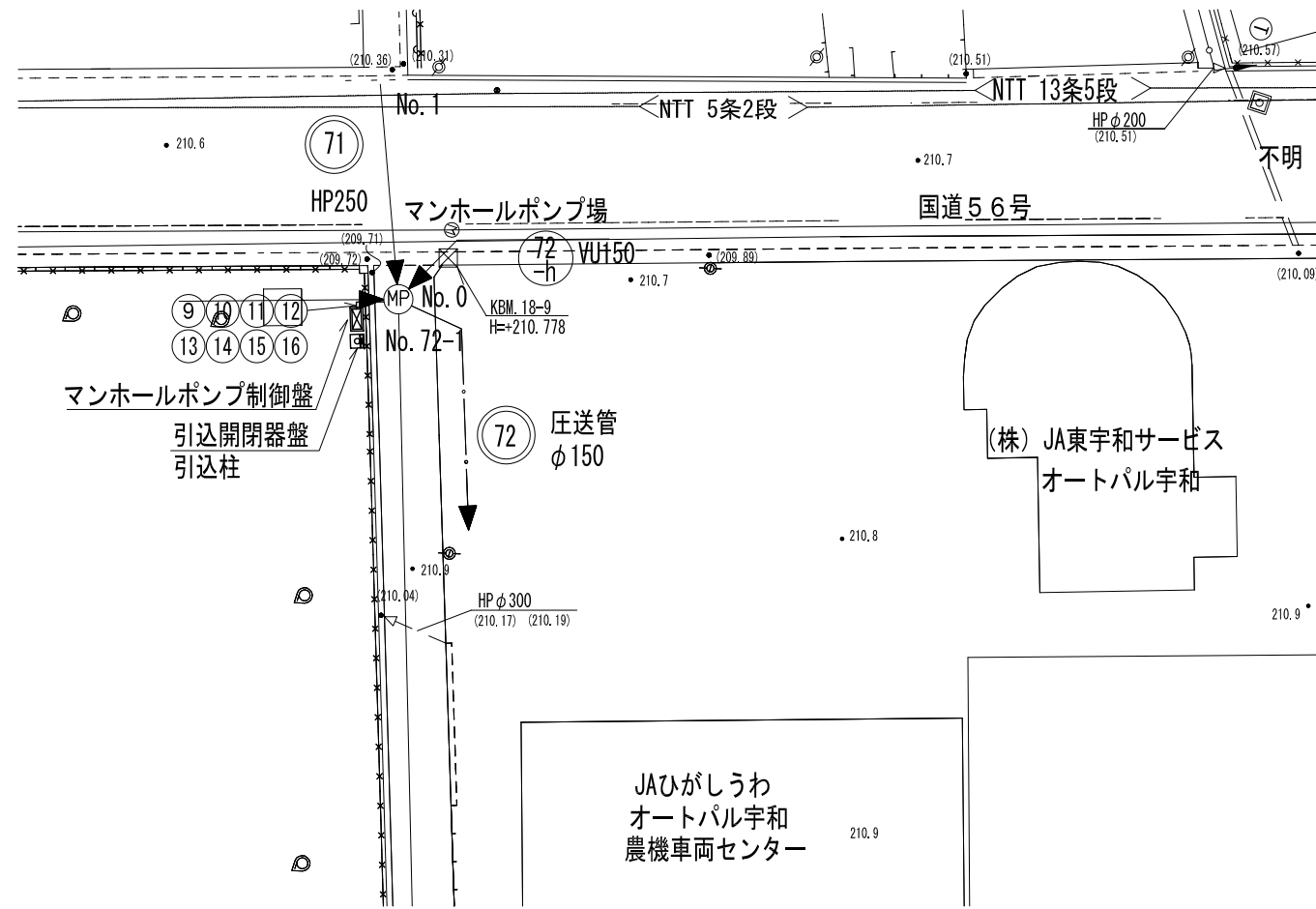
マンホールポンプ全体配置平面図
